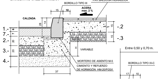
ENCUENTRO CALZADA-ACERA
